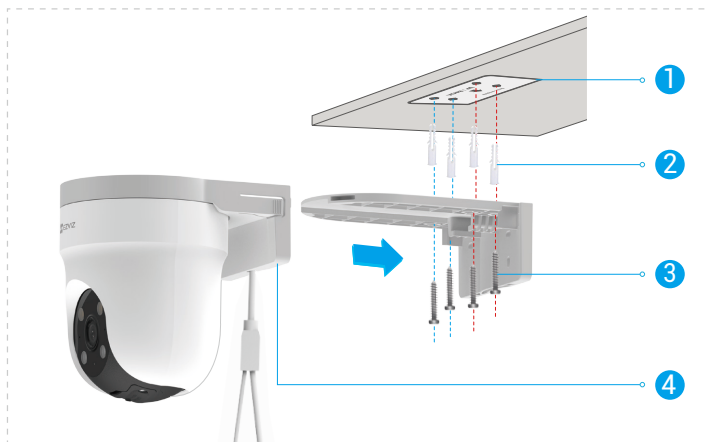
Рисунок 1. Монтаж на потолок
