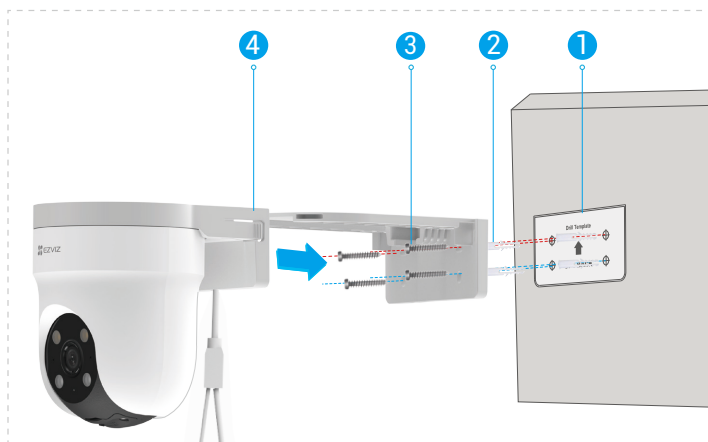
Рисунок 2. Монтаж на стену
